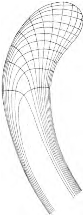
Fig. 319. Gebogener Krahn mit Zug und Druckkurven. Nach einer Konstruktion von CULMANN aus H. V. MEYER.
